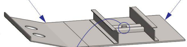
Conj. Mesa Simples Inclinada c/ Pino Rei Soldado 19.054
