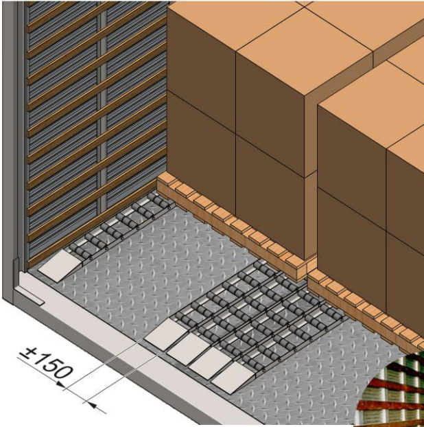
CJ Piso Roletado TPI Fixo - 411.003
